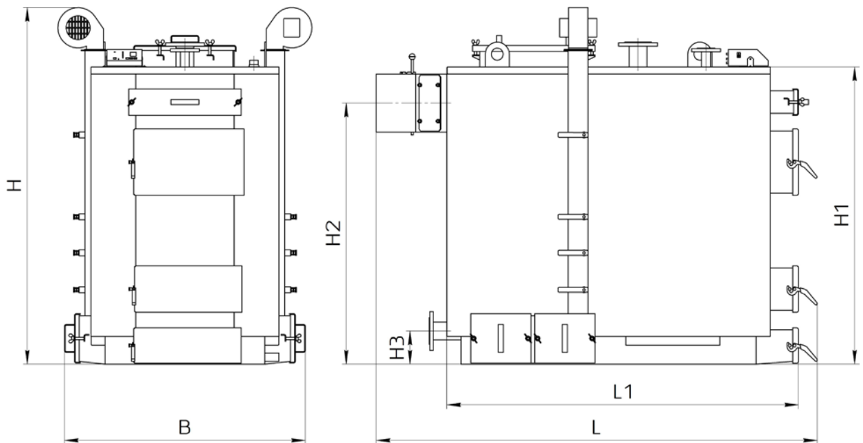
Рисунок 1 – Габаритне креслення котла типу КТ-3Е
