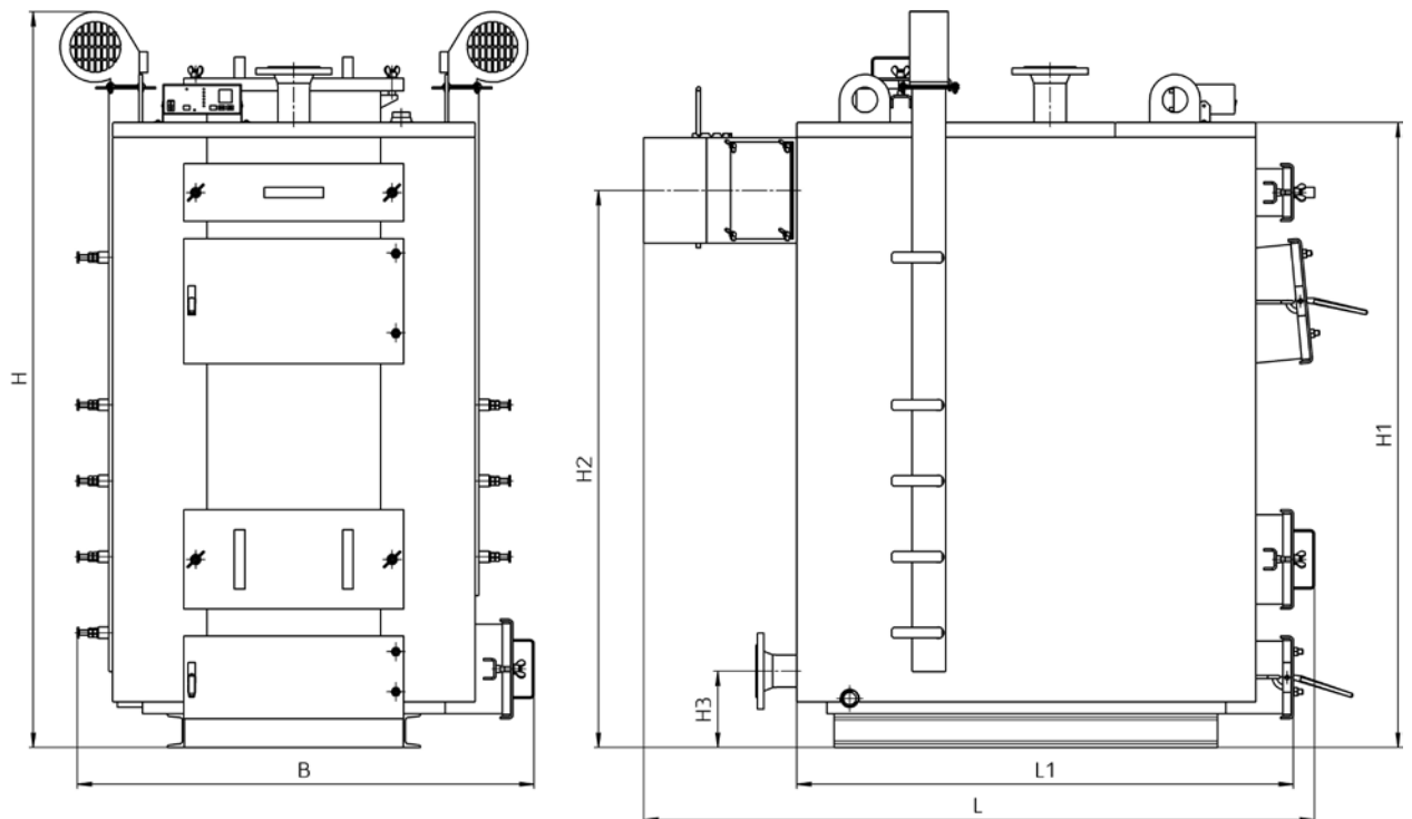
Рисунок 1 – Габаритне креслення котла типу КТ-3Е
